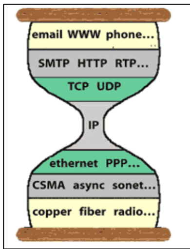
Figure 21-2. IETF Hourglass
